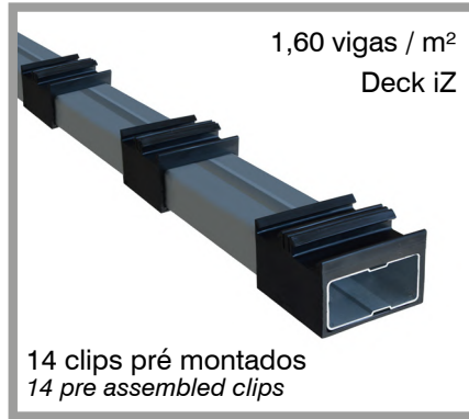
IZ Viga Aluminio c/ Clips pré montado Beam • Lambourde • Unterstruktur • Viga
